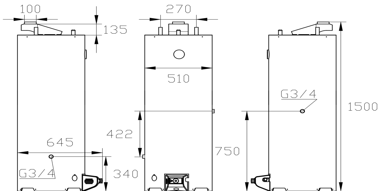
Рис. 5 Габаритные и присоединительные размеры НГВ ТЕПЛОПУС 120 л
