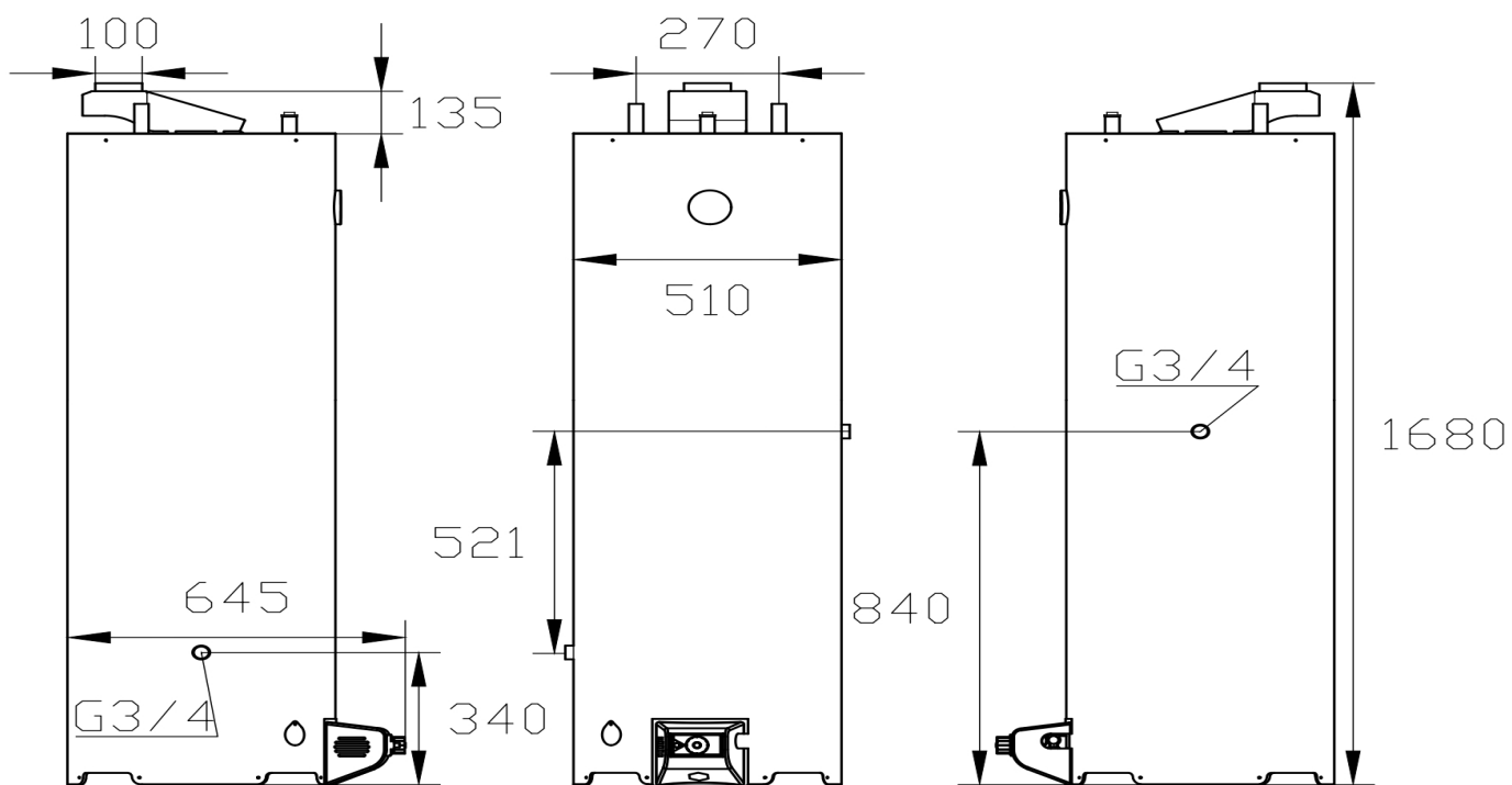
Рис. 7 Габаритные и присоединительные размеры НГВ ТЕПЛОПУС 190 л
